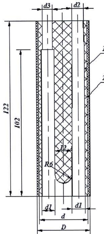
Hình 1 - Mồi nổ dùng cho thuốc nổ công nghiệp
