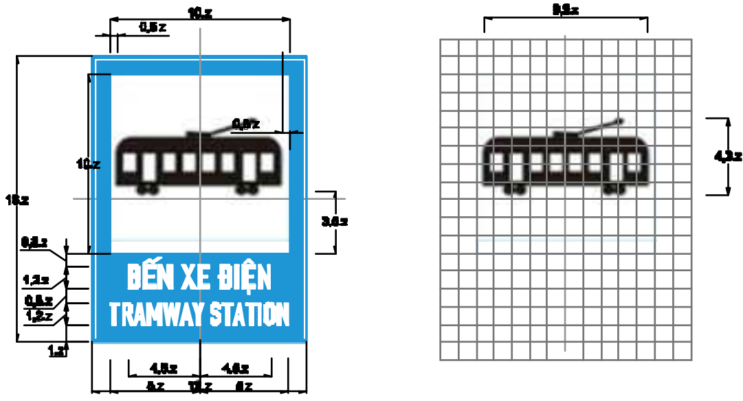
Biển số L435 : Bến xe điện
