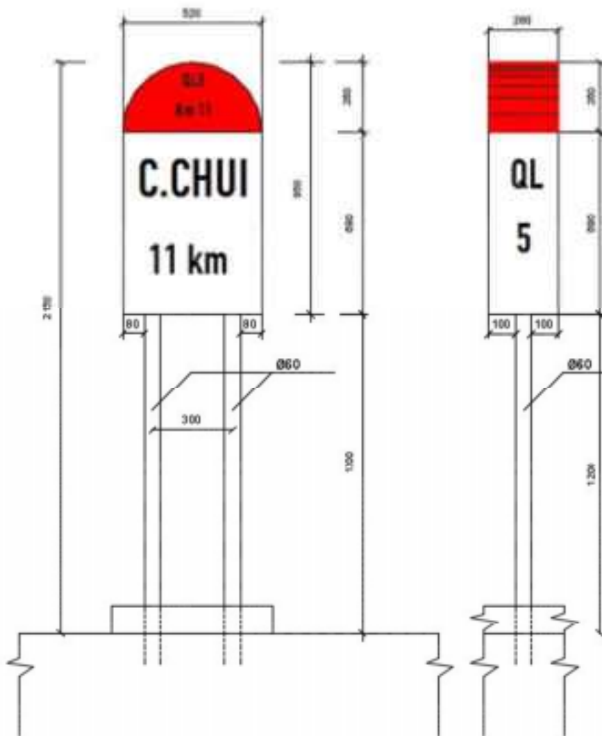
Ghi chú: Kích thước ghi trên hình vẽ là mm Hình I.2 - Cột kilômet dạng cột cao
