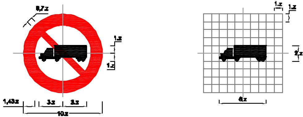
Biển số P.108a: Cấm xe sơ-mi-ro-móc
