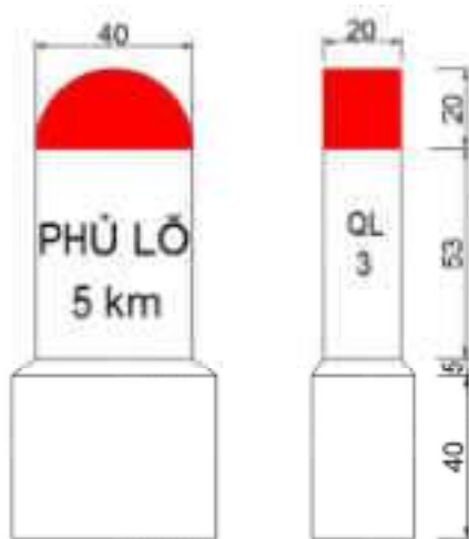
Ghi chú: Kích thước ghi trên hình vẽ là cm Hình I.1 - Cột kilômet dạng cột thấp
