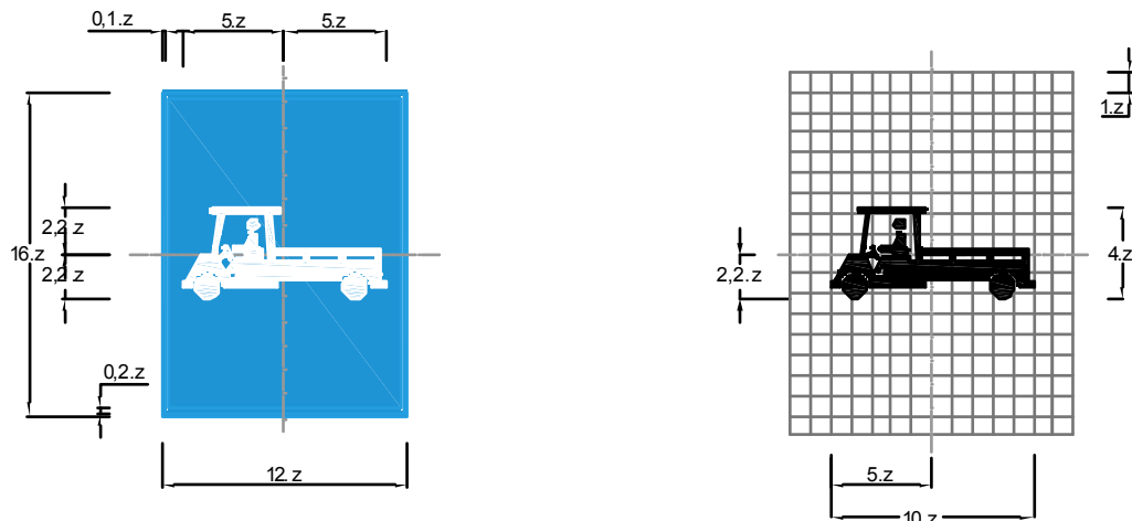
Biển số R.403h: Đường dành cho xe chở người bốn bánh gắn động cơ
