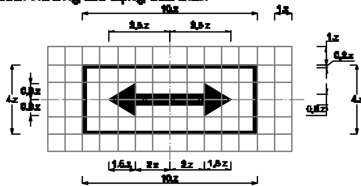
Biển số S.503c: Hướng tác dụng của biển
