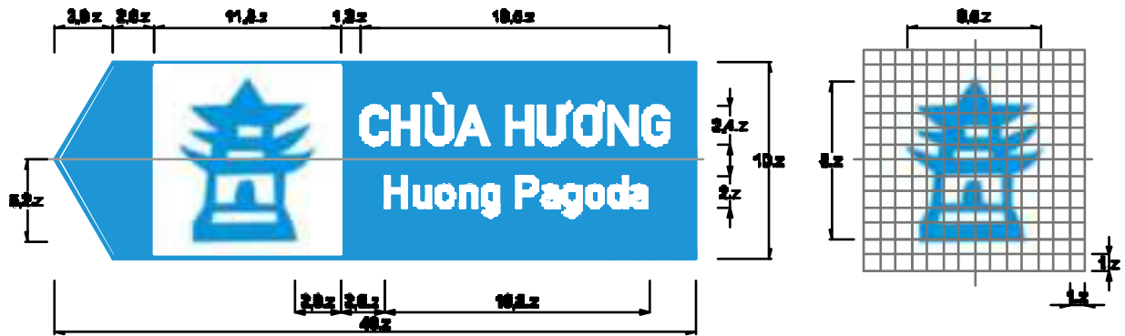
Biển số L.444g : Biển báo chỉ dẫn địa điểm
