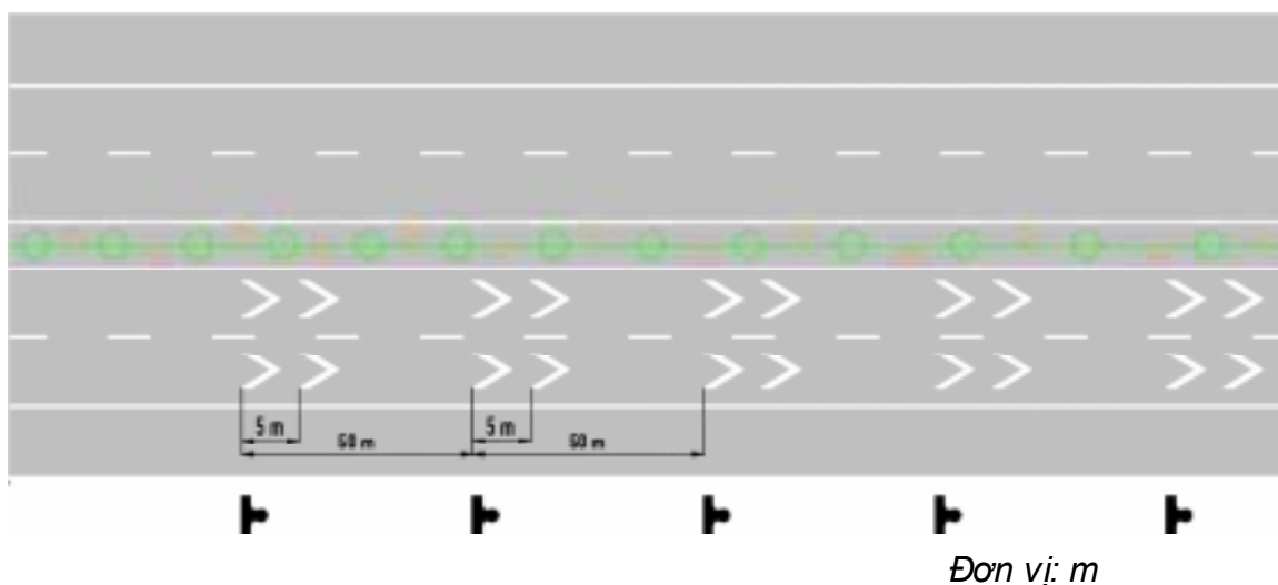
Hình G.57 - Bố trí vạch h xác định khoảng cách xe trên đường
