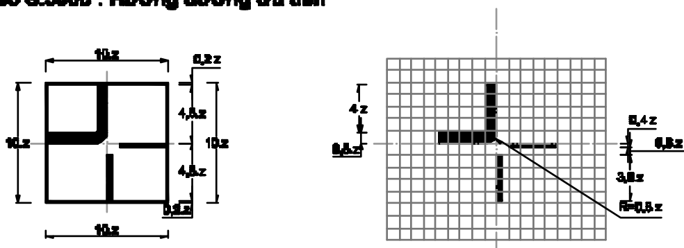
Biển số S.506b : Hướng đường ưu tiên
