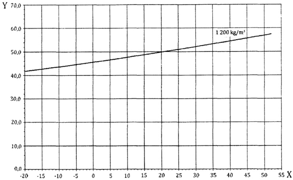
Hình 3 — Đồ thị nhiệt độ/áp suất đối với FK- 5-1-12 được nén cực đại bằng nitơ đến 42 bar ở 20°C
