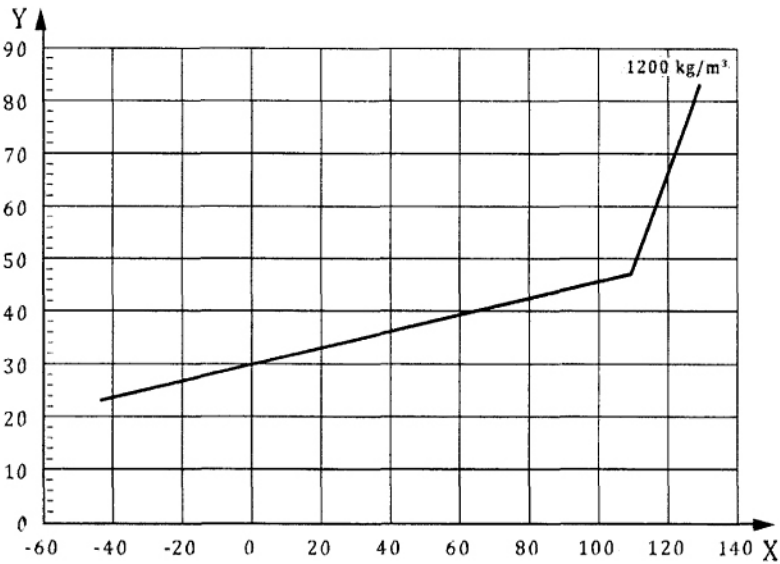
Hình 1 — Đồ thị nhiệt độ/áp suất đối với FK- 5-1-12 được nén cực đại bằng nitơ đến 25 bar ở 20°C
