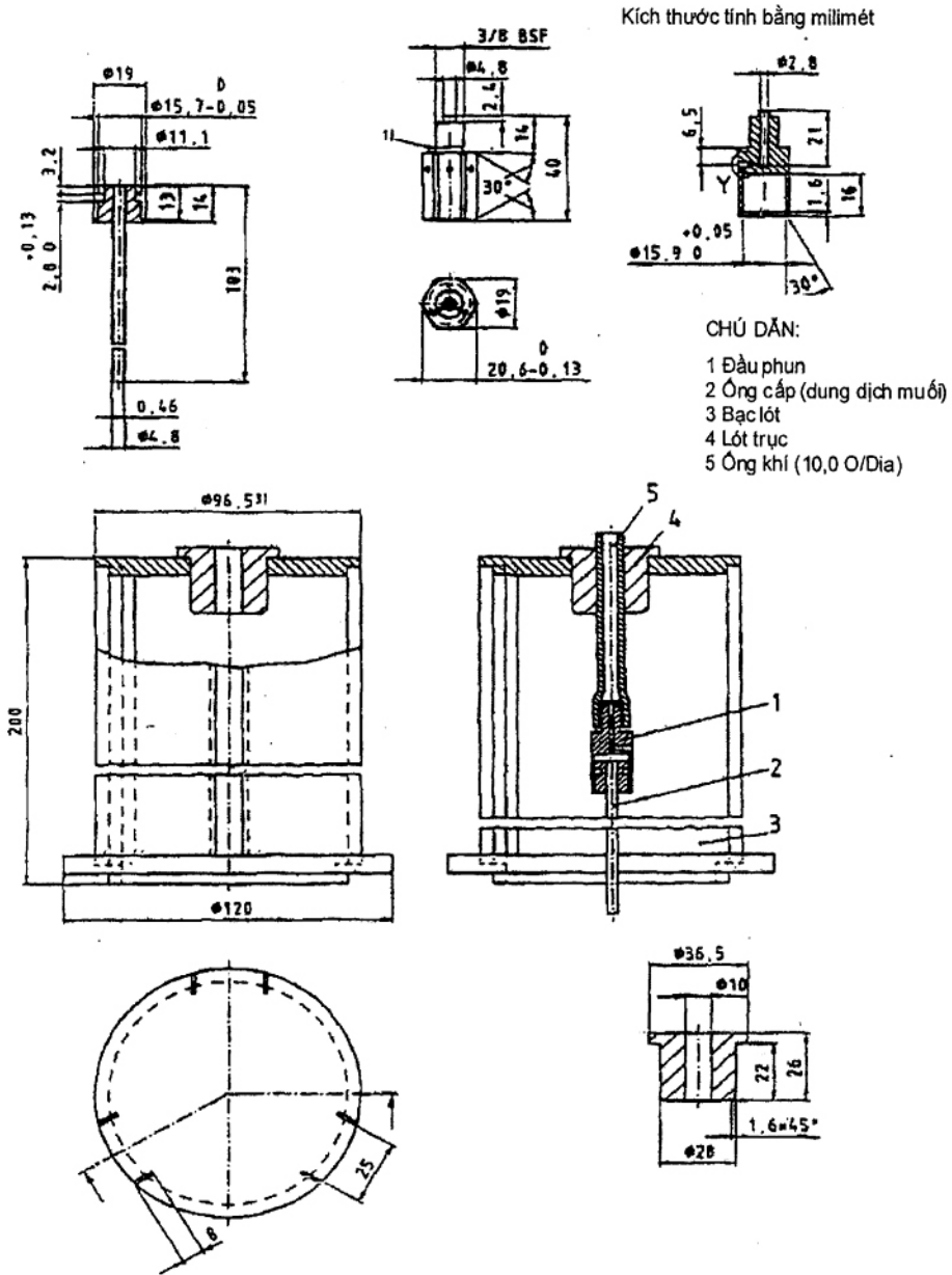
Hình 13 - Cách bố trí máy phun
