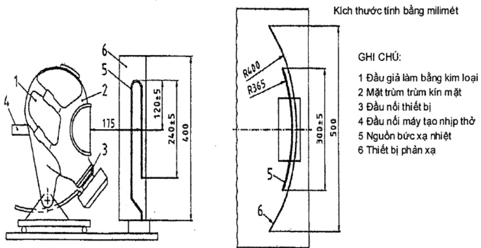
Hình 4 - Sơ đồ thử nghiệm khả năng chịu bức xạ nhiệt
