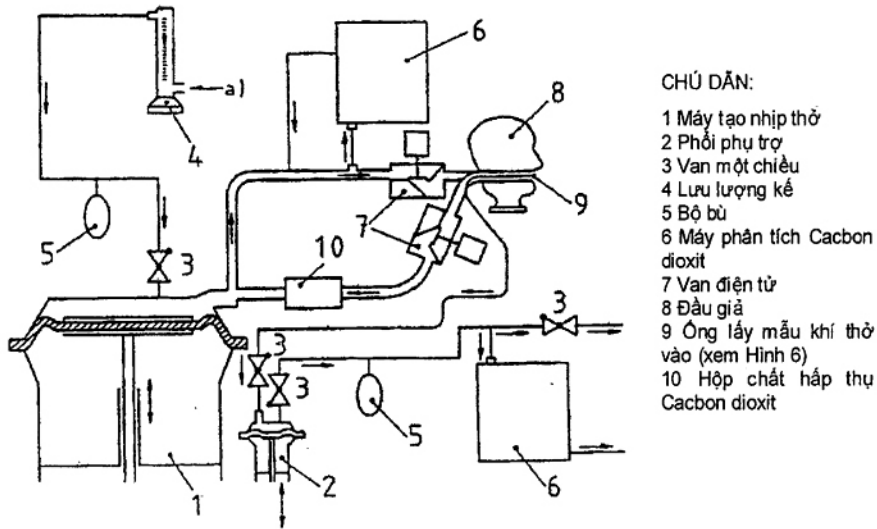
Hình 7 - Sơ đồ hệ thống thử nghiệm hàm lượng Carbon dioxide trong khí thở vào
