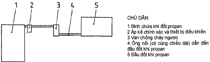
Hình 3 - Sơ đồ thử nghiệm tính bắt cháy của mặt trùn loại 2 và loại 3
