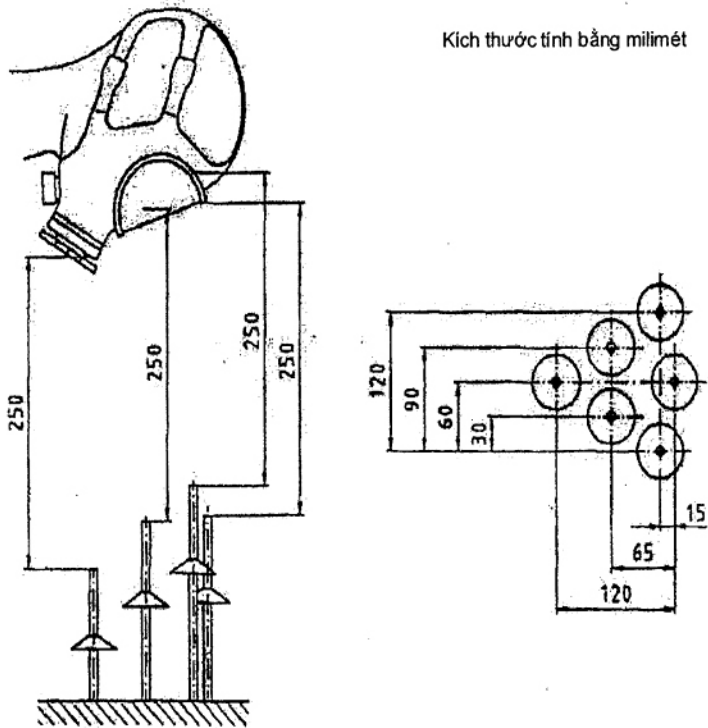
Hình 2 - Sơ đồ bố trí đầu đốt khí propan
