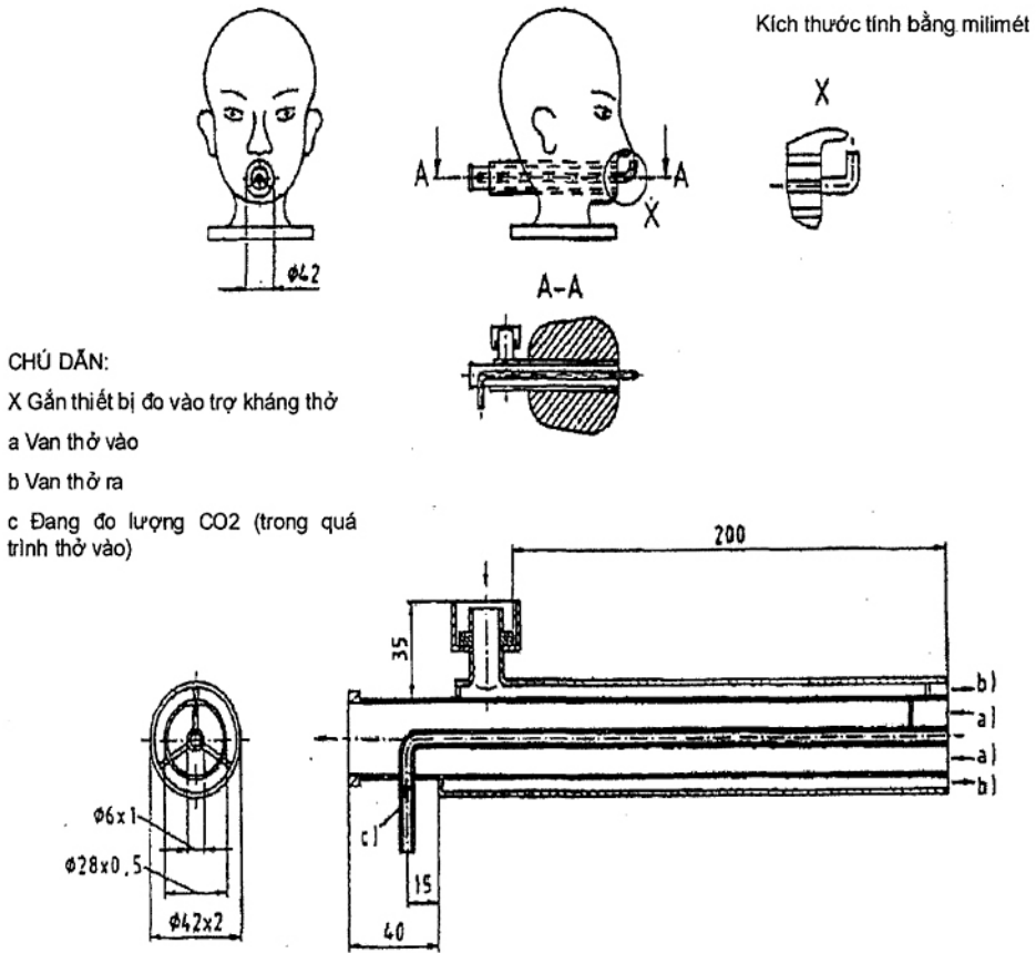
Hình 6 - Đầu giá Sheffield để thử nghiệm hàm lượng Cacbon dioxit trong khí thở vào (không gian chết) và trở lực hô hấp của mặt trùm.
