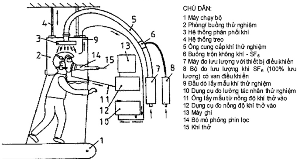
Hình 10 – Sơ đồ bố trí hệ thống kiểm tra rò rỉ khí bên trong dùng lưu huỳnh hexaflorit
