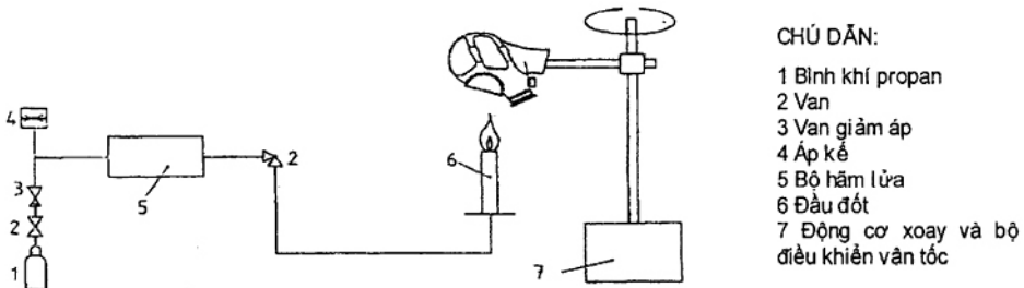
Hình 1 - Sơ đồ thử nghiệm tính bắt cháy của mặt trùm loại 1
