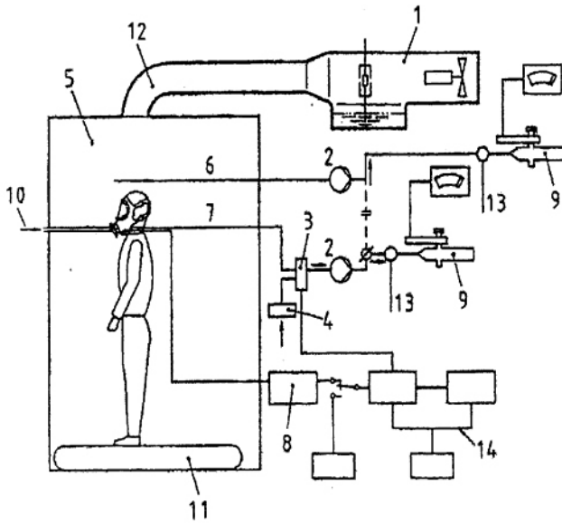
Hình 12 – Sơ đồ sắp xếp hệ thống để kiểm tra rò rỉ khí vào bên trong sử dụng NaCl
