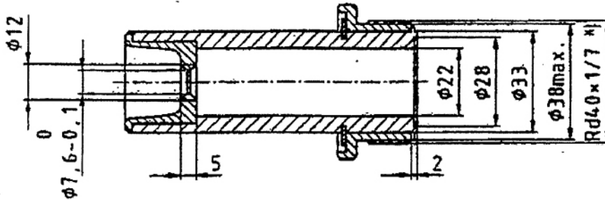
Hình 9 – Bộ phận thiết bị lọc mô phỏng dành cho mặt trùm/ thiết bị lọc sử dụng một ren vít theo EN 148-1
