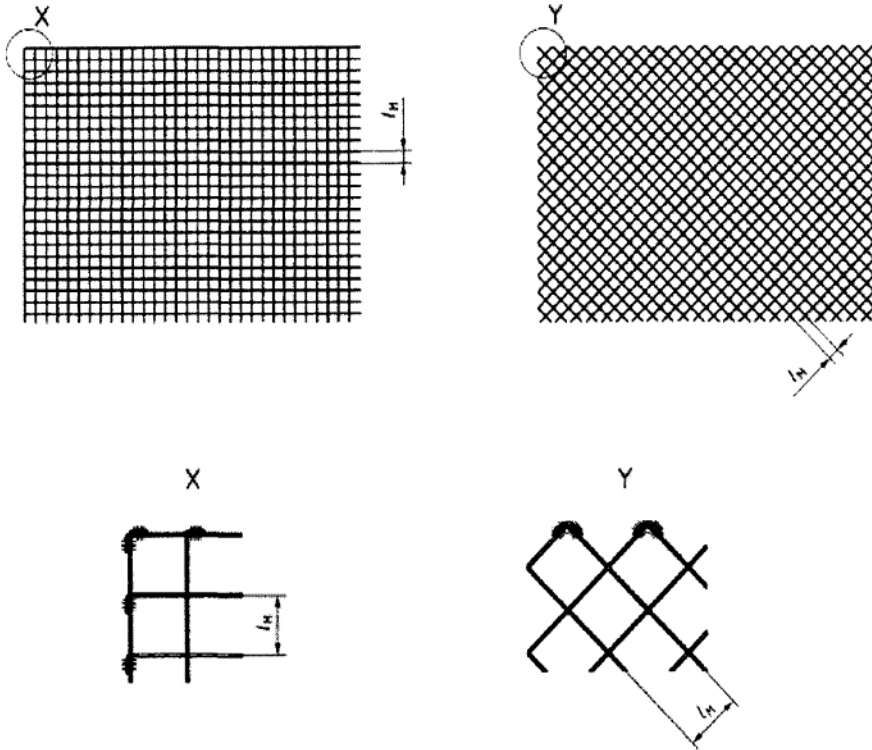
a) Tổ hợp mắt lưới hình vuông (Q)
