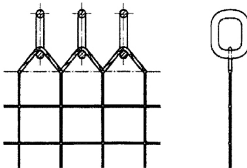
Hình 11 – Sơ đồ cố định lưới vào khung ống (sơ đồ nguyên lý)
