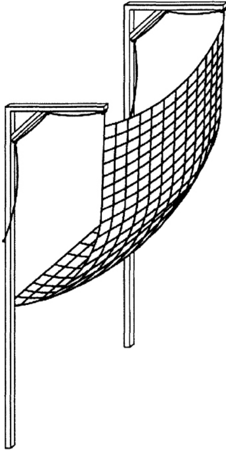
Hình 4 - Hệ thống lưới an toàn V (lưới với dây biên treo vào giá đỡ kiểu khung công xon)
