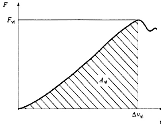
Hình 12 – Đồ thị lực kéo giãn dài của các mắt lưới chịu phong hóa
