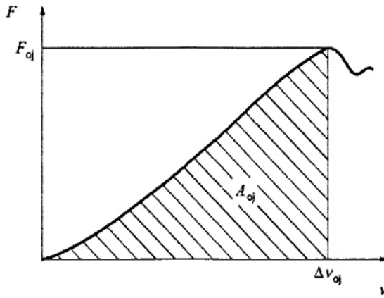
Hình 13 – Đồ thị lực kéo giãn dài của các mẫu mắt lưới ở trạng thái như mới
