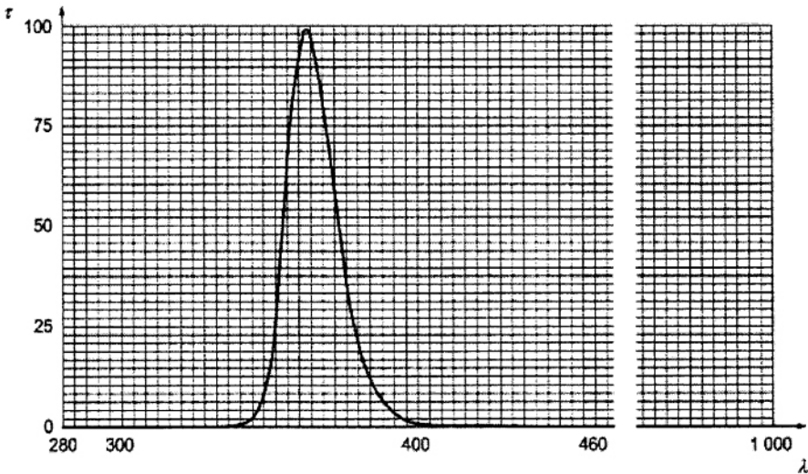
Hình 14 – Bộ lọc bức xạ dải bước sóng từ 300 đến 420 nm
