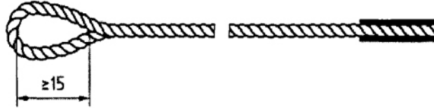
d) Dây lưới N (dây nối)
