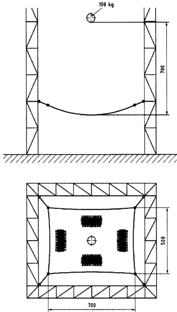
Hình 18 - Thử nghiệm và đập hệ thống lưới an toàn S
