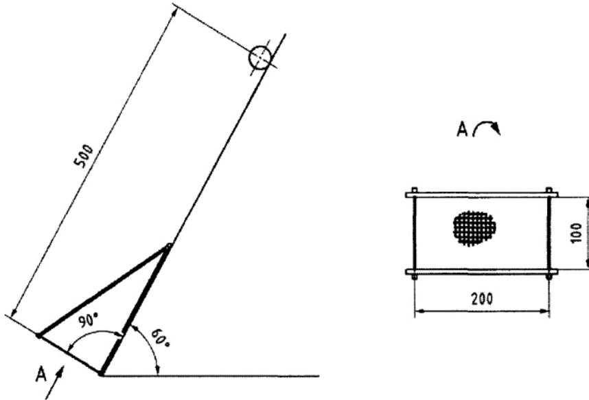
Hình 20 – Mặt dốc nghiêng thử nghiệm hệ thống lưới an toàn U
