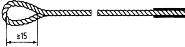
b) Dây lưới L và F (dây buộc, sử dụng đơn với chỉ một đường kính chịu tải) Dây lưới R và dây lưới H (dây buộc, sử dụng đôi với hai đường kính chịu tải)
