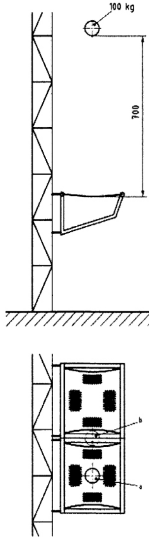
Hình 19 - Thử nghiệm độ bền động của hệ thống lưới an toàn T
