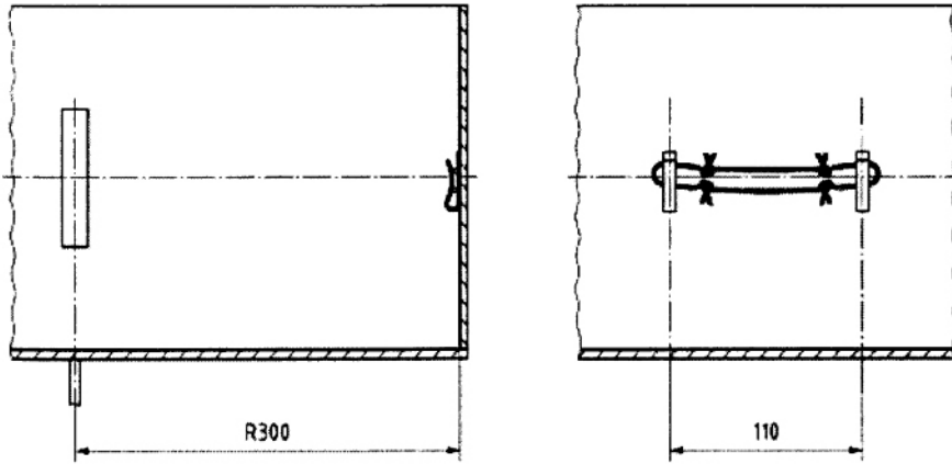
Hình 16 - Vị trí các mẫu thử trong buồng thử nghiệm phong hóa nhân tạo
